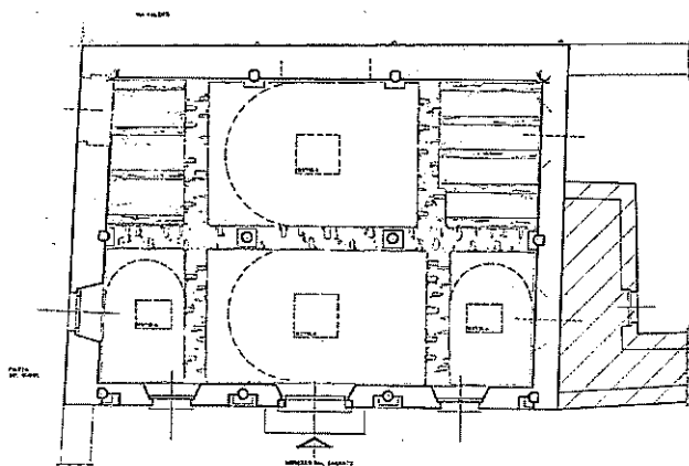
fig. 2 - Pianta delle volte esistenti sotto "Sala Colonne".
